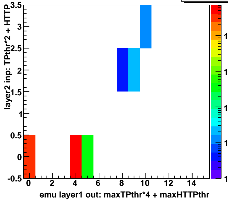
TP (+) HTTP thres, JP_Falk(3+4+5), trig=allTrig
