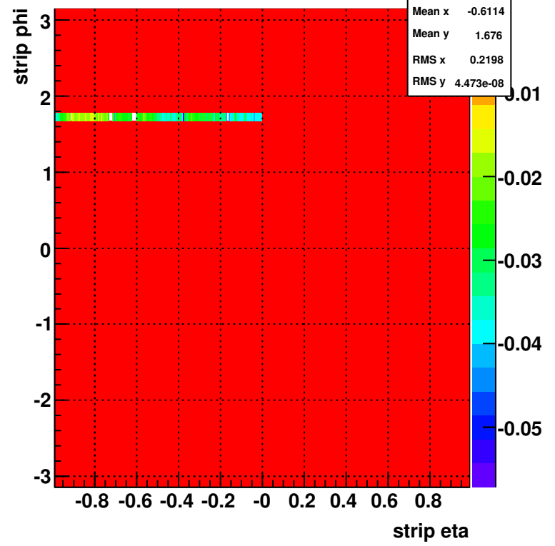
bsmdp slope vs. eta and phi
