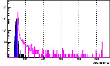
BSMD Strip 520_e
