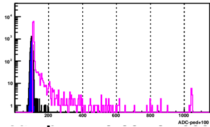
BSMD Strip 778_e
