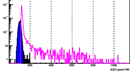
BSMD Strip 1489_e
