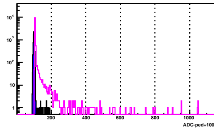
BSMD Strip 641_e
