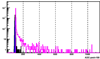
BSMD Strip 658_e
