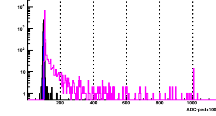
BSMD Strip 209_p
