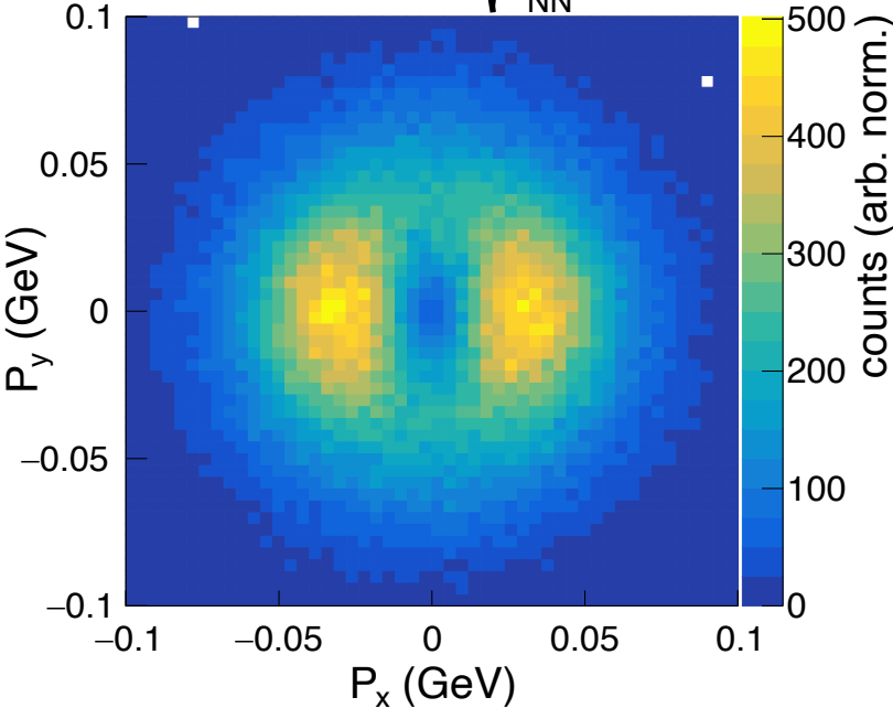
C STAR: Au+Au at \sqrt{s_{NN}}=200 GeV
