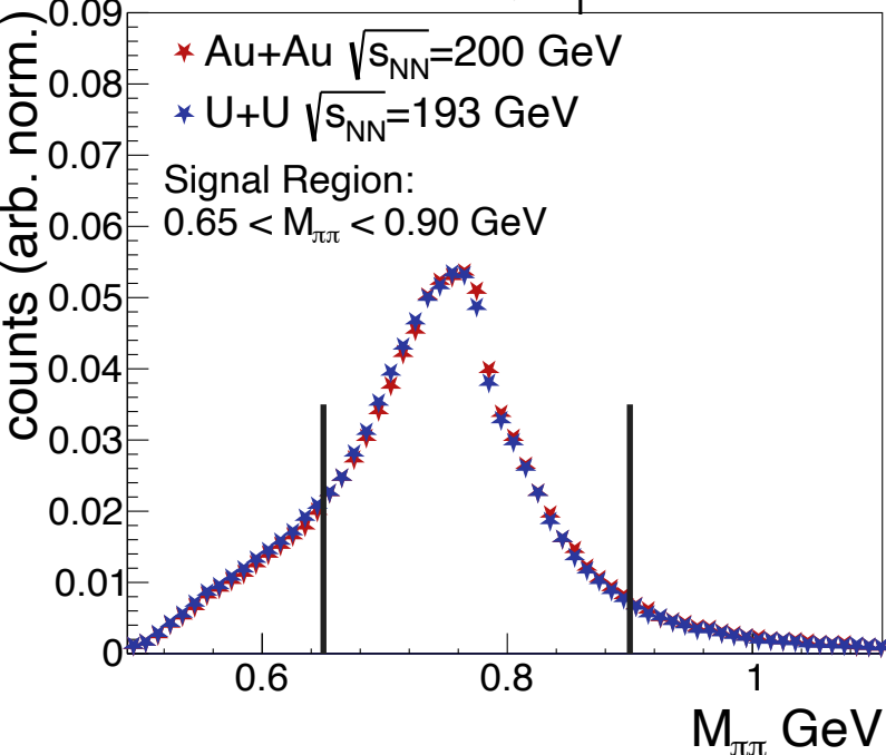
C STAR: Au+Au at \sqrt{s_{NN}}=200 GeV
