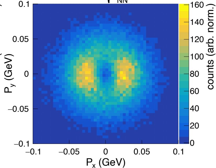
D STAR: U+U at \sqrt{s_{NN}}=197 GeV
