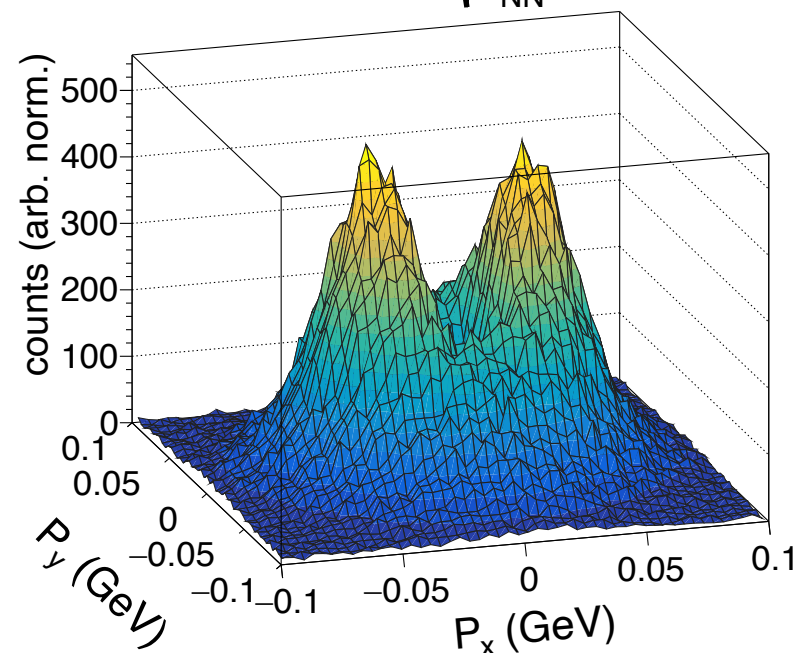
B STAR: Au+Au at \sqrt{s_{NN}}=200 GeV
