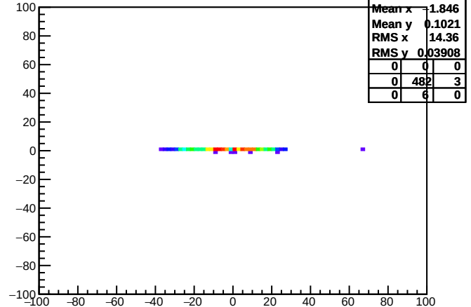
StE VPD vtxz vs TPC vtxz
