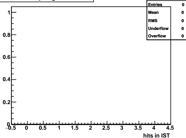
StE IST: Hits per global track
