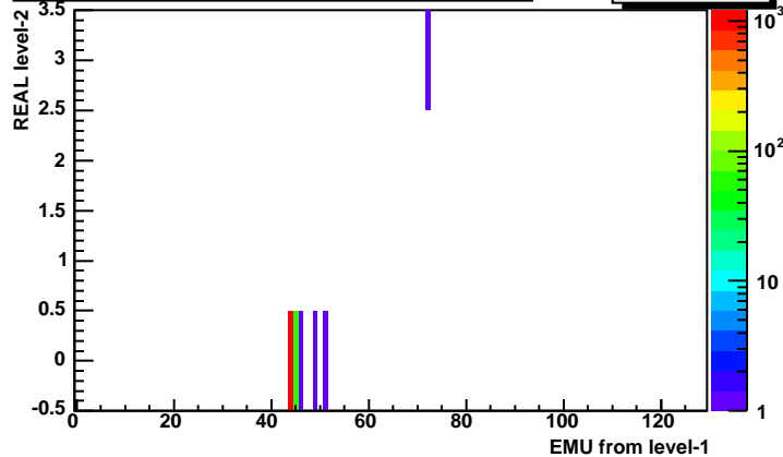
TP inp vs. emu, layer-2, JP_Falk(4), trig=allTrig
