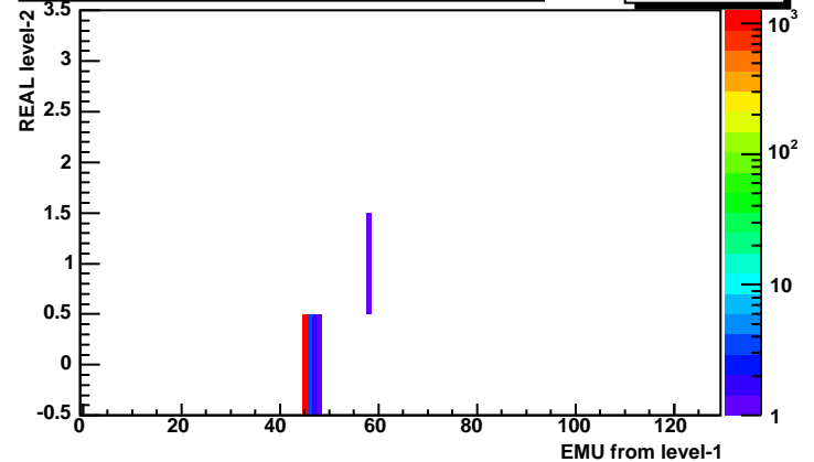
TP inp vs. emu, layer-2, JP_Falk(5), trig=allTrig
