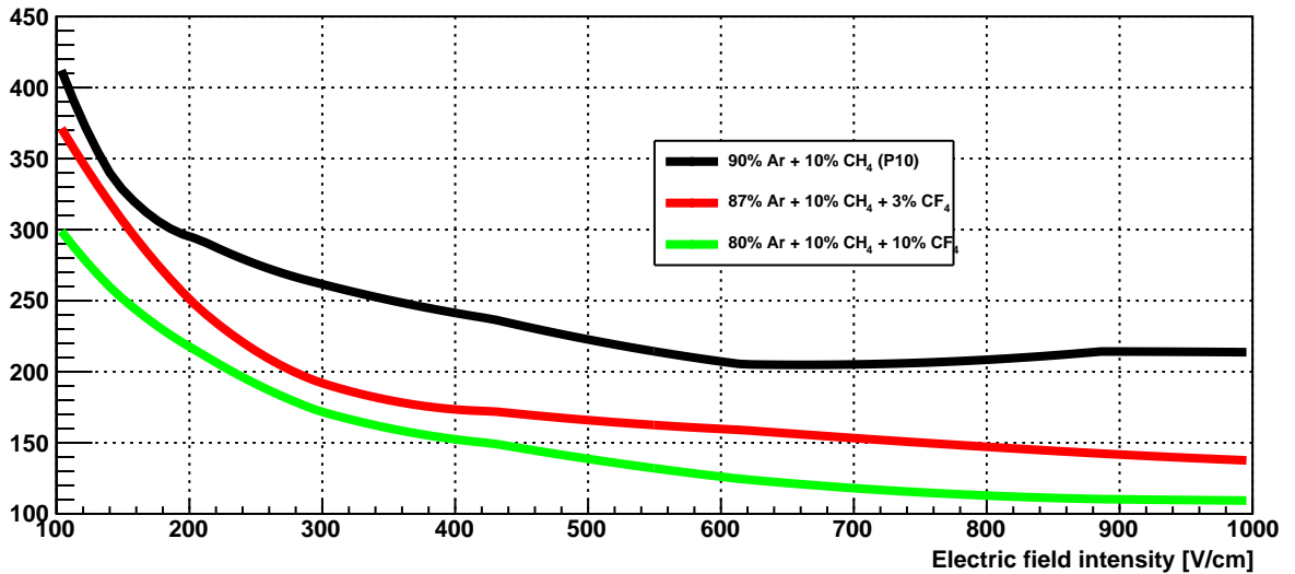
Electron longitudinal diffusion [ \mu m/ \sqrt cm]
