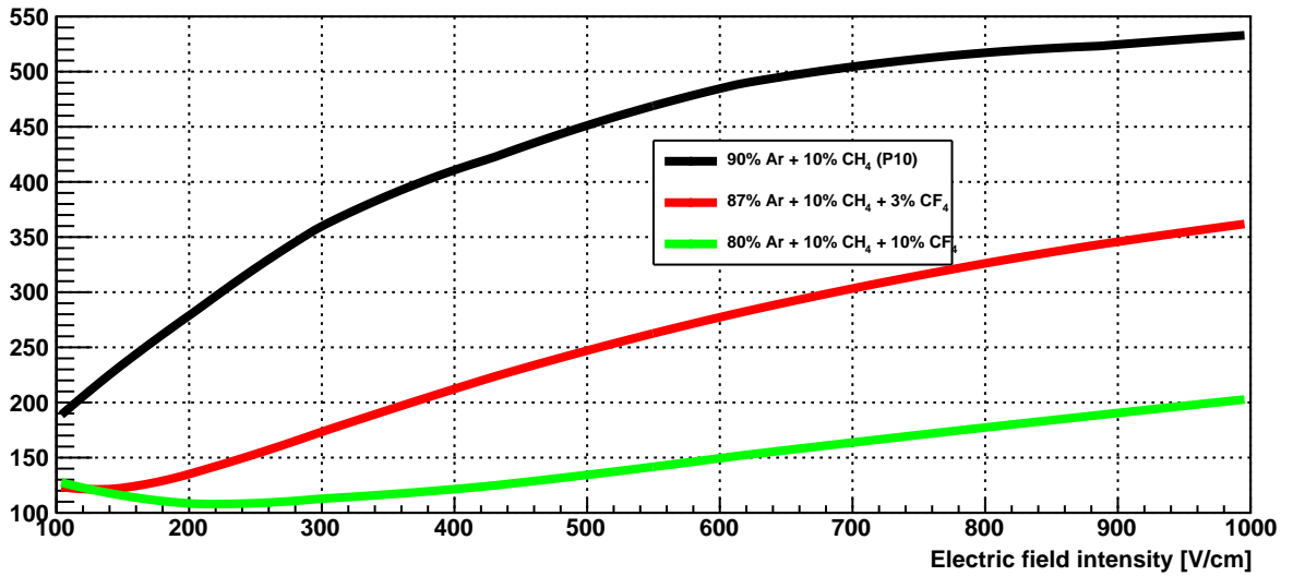
Electron transverse diffusion [ \mu m/ \sqrt cm]
