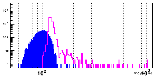
BSMD Strip 2935_e
