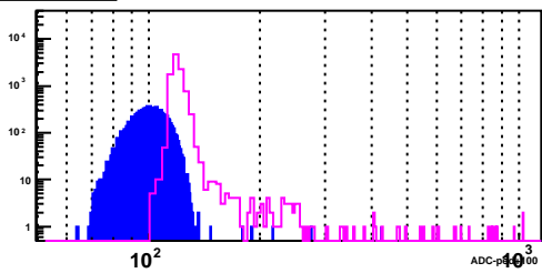
BSMD Strip 2936_e
